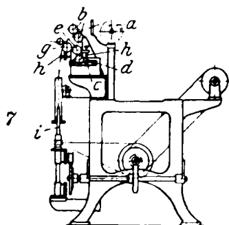
Ringspinnmaschine (f) für Papiergarn ring spinning machine for paper yarn кольцепрядильный ватер (мр) для бу- мажной пряжи métier (m) à filer à anneau pour fil de papier filatoio (m) continuo ad anelli per filo di carta máquina (f) de hilar de anillos para hilos de papel / máquina (f) de hilar d'anells per a fils de paper
