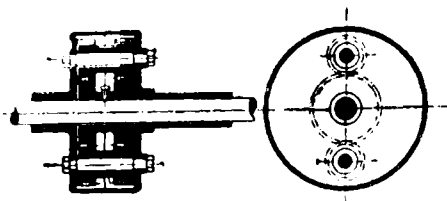
Brooks u. Doxey's Differentialgetriebe (n)
