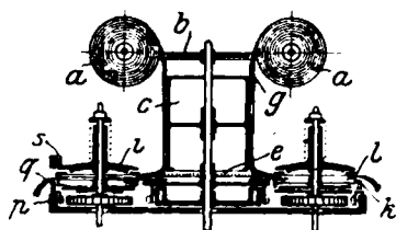
Lustersche zwei- köpfige Seiden- kämmaschine (f)
