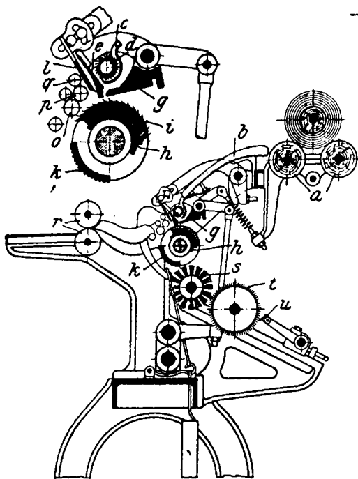
Heilmann'sche Kämmaschine (f)
