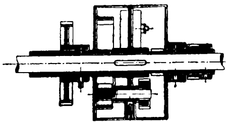
Stirnrad differentialwerk (n) mit doppelter Übersetzung spur wheel differential motion with double gearing
