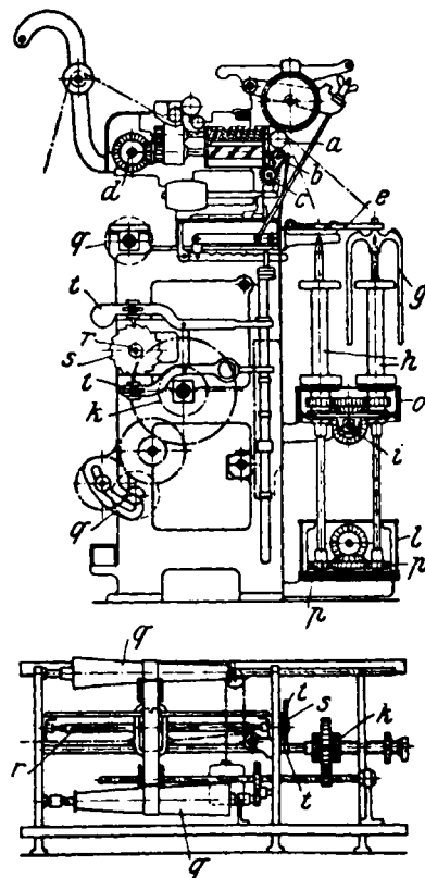
Jutevorspinnmaschine (f) jute roving frame баннаброш (мр) для джута banc (m) à broches pour jute 13 banco (m) a fusi per juta mechera (f) para yute / me- txera (f) per a jute
