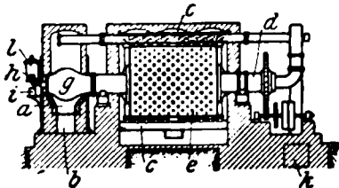
Auskohler (m) [oder Karbonisiervorrichtung (f)] f6r Lumpen carbonising apparatus for rags карбонизационное устройство (ср) для лоскута carboniseuse (f) pour chiffons apparecchio (m) di carbonizzazione per stracci carbonizador (m) de trapos / carbonitzador (m) de draps
