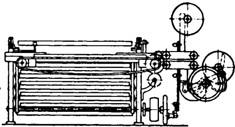
Anstückelmaschine (f) machine (f) pour former une mèche continue
