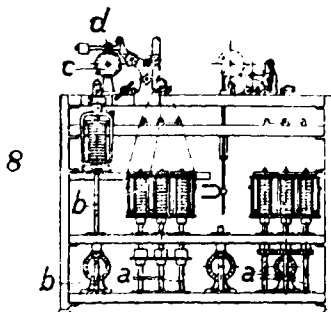
Litzenaustreib- maschine (f), Litz- zwirnmaschine (f), Verlitzmaschine (f), Kordelmaschine (f) twine laying machine, strander, stranding machine, twine layer, cabling ma- chine, register[ing] machine машина (жр) для производства или скручивания стренг machine (f) à fabriquer les torons, toron- neuse (f) macchina (f) per fare trefoli máquina (f) de fabricar cordeles / cordills
