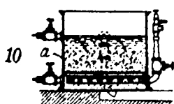
Kiesfilter (n) gravel filter фильтр (мр) из гравия filtre (m) à gravier filtro (m) a ghiaia filtro (m) de grav[ill]a / filtre (m) de grava o de sorra granada
