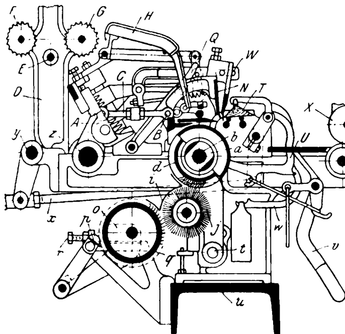
Nasmith's Kämmaschine (f) Nasmith's comb гребнечесальная (жр) Не- смита peigneuse (f) Nasmith pettinatrice (f) Nasmith peinadora (f) / pentinadora (f) / Nasmith
