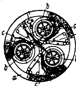
Noblesche Kämmaschine (f) Noble's comb[er] гребнечесальная (жр) системы Нобля peigneuse (f) Noble pettinatrice (f) tipo Noble peinadora (f) / pentinadora (f) / Noble
