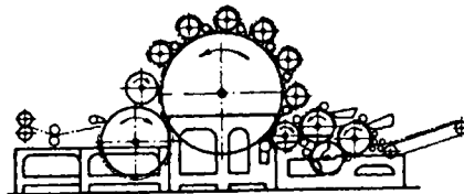
einfache Kammgarnkrempe (f)
