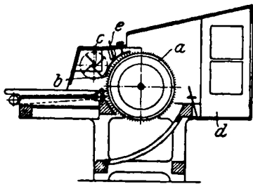
Lumpenreißmaschine (f) rag grinder, rag devil лоскуторазрывная машина
