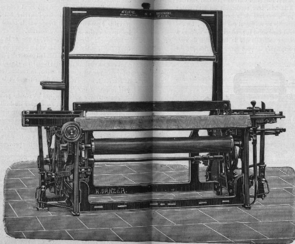
FIG. 73. — Métier mécanique, Diderichs de Bourgoin.
