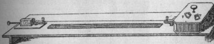
FIG. 49. — Compteur d'apprêts, d'après Pariset, Monographie de l'industrie de la soie (Bulletin des soies et des soieries).
