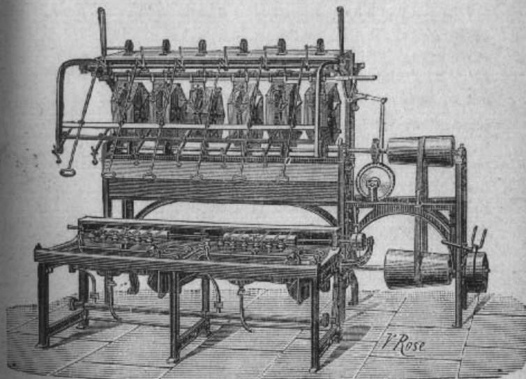
FIG. 38. — Appareil à filer la soie à deux bassines, système Léon Camel, construit par les chantiers de la Buire à Lyon.
