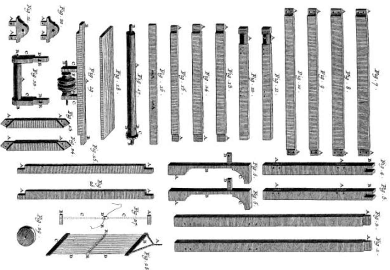
Passementerie, détail du Miter à Françoise
