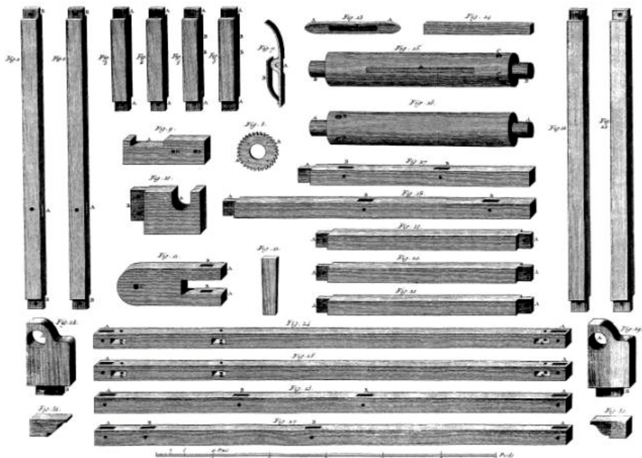
Détail des Pièces du Mûrier à Marly.
