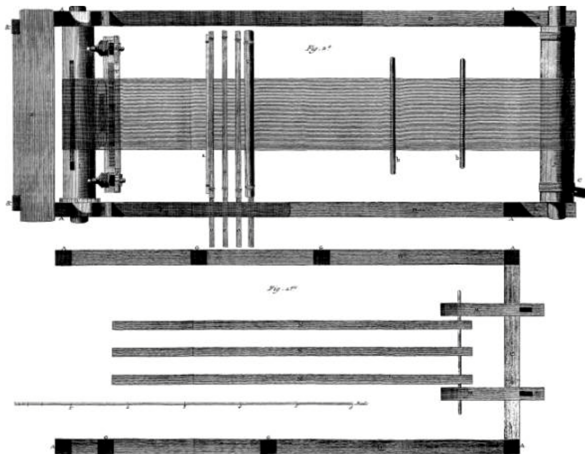
Plans du Métier à Marly.
