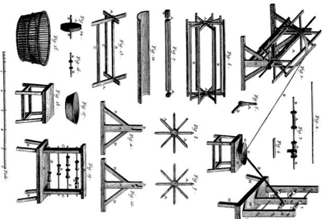
Passementerie, Détails des Outils propres à faire le Nonpareille.
