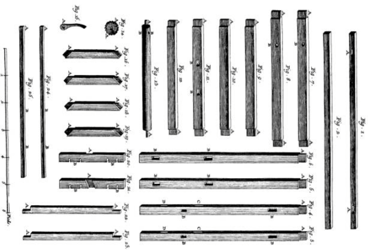
Passementerie, Détails du Moutre à la Rayée Lisse.
