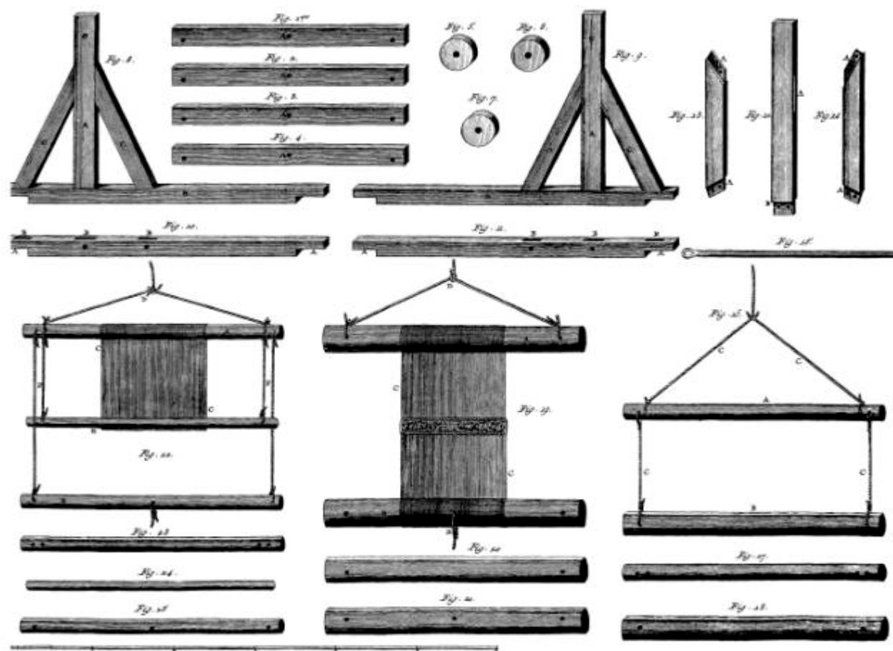
Détail des Pièces du Métier à Marly.
