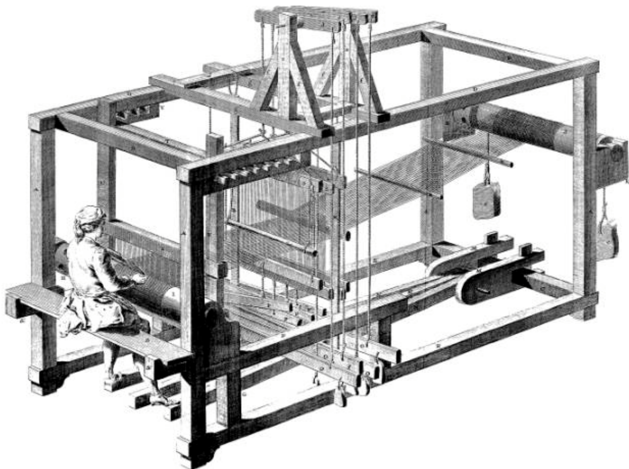
Métier à Marly.
