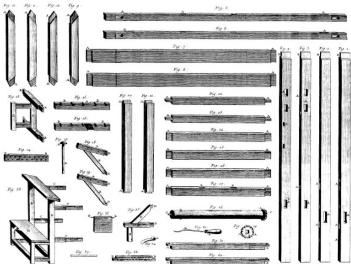
Passementerie, détail du Métier à faire le Galon.
