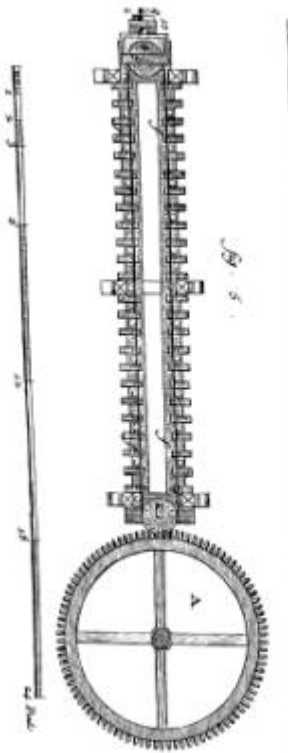
Fil, Moulin Quarté.
