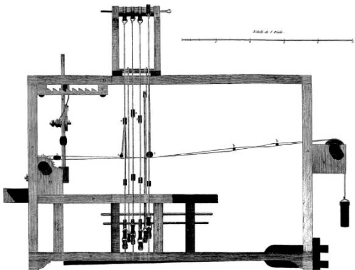
Élévation Latérale Du Mètier à Marli.
