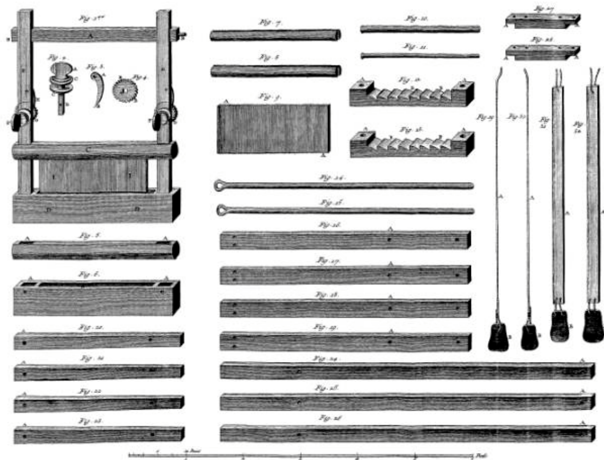
Détail des Pièces du Mûrier à Marli.
