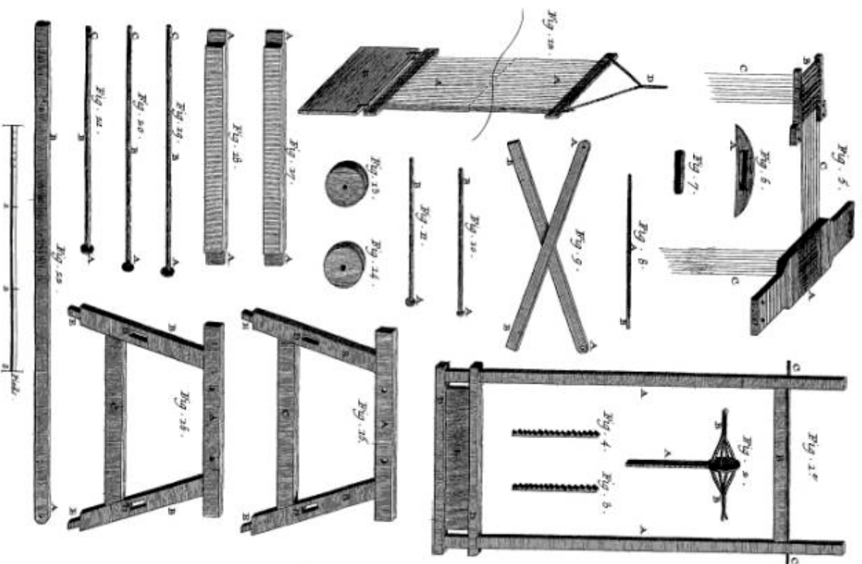
Passementerie, Détail du Mètre à tison.
