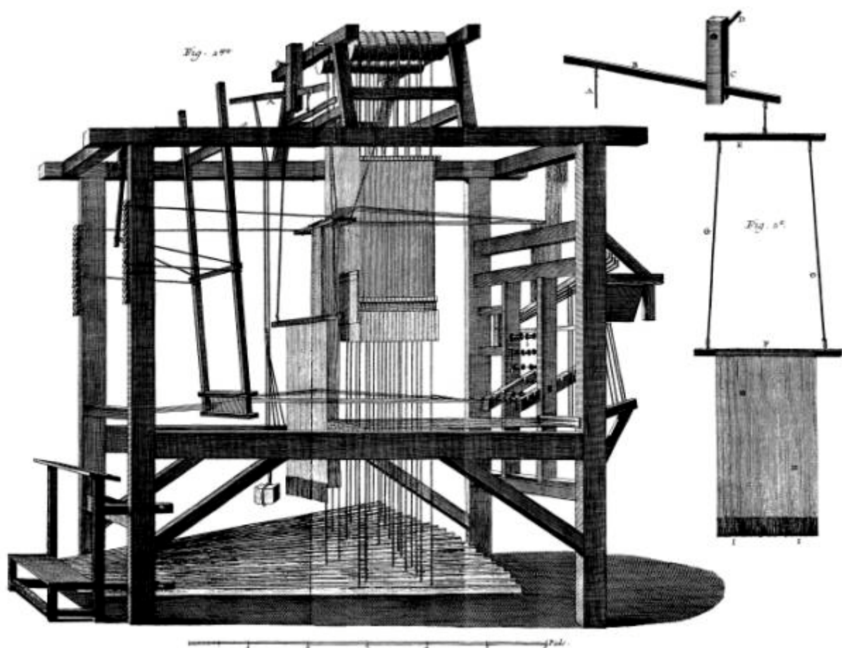
Passementerie, Métier du Ruban figure 2.
