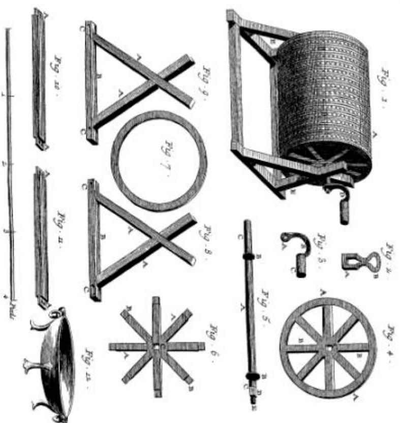
Passementerie, Pompage du carton.
