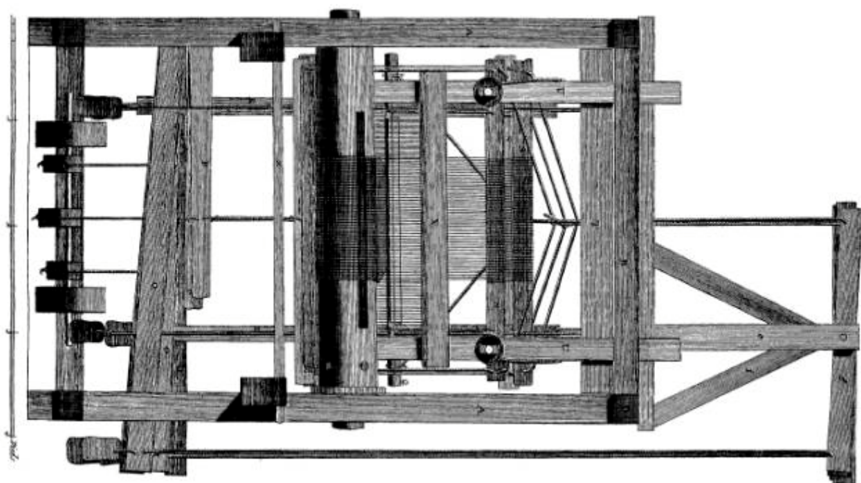
Élévation en face Du Mètier à Marli.
