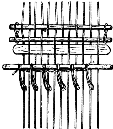
FIG. 40.—Headle Rod.
