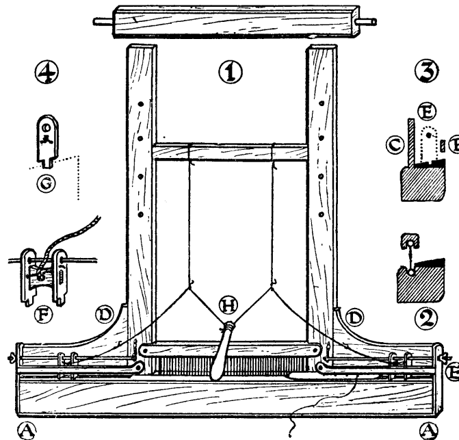
FIG. 54.—Fly-shuttle Batten.
