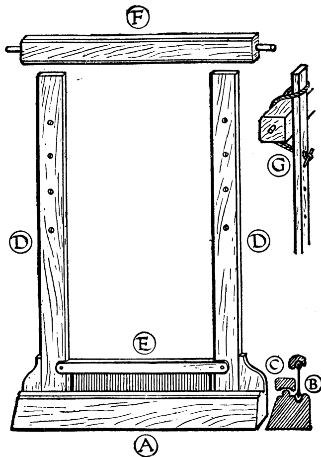
FIG. 46.—Hand-batten.
