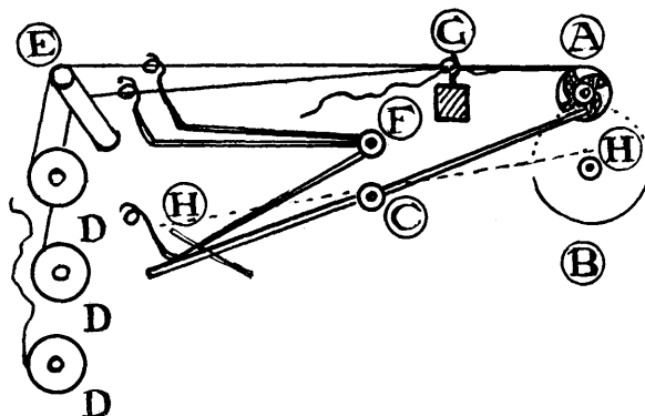
FIG. 17. DOUBLER
