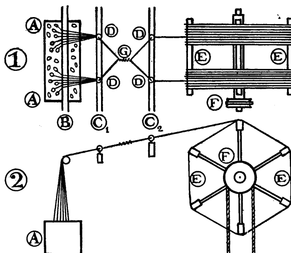
FIG. 13. REELING MACHINE
